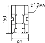
③ Колонна задняя
