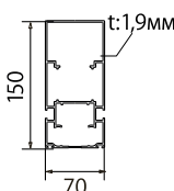
② Несущая балка со сливным лотком
