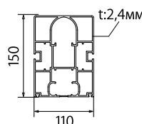
④ Монтажный профиль
