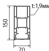
③ Колонна фронтальная
