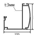
② Несущая балка со сливным лотком
